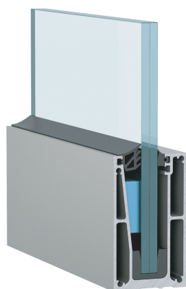
Sistema Slim Line portata 200Kg.
