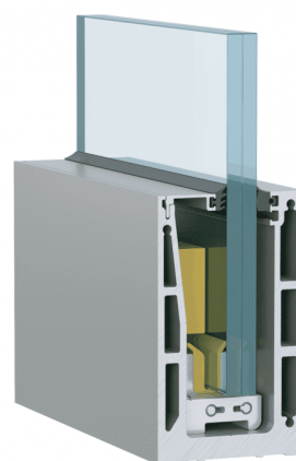
Sistema L Line portata 300Kg.
